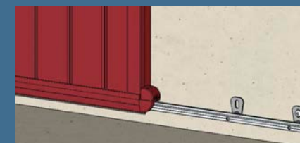
Réglette support en partie basse pour porte-fenêtre
