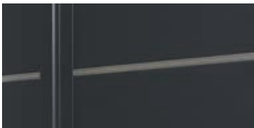
Galet emprisonné sur rail anti-déraillement.
